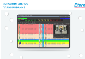
Этере Scheduling
